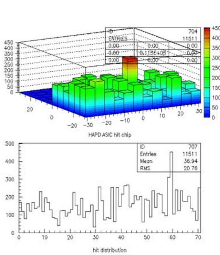
図 4.40: HAPD+ASIC で得られた HAPD の Hit 情報
