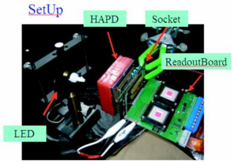
図 4.37: HAPD+ADIC の SetUp
