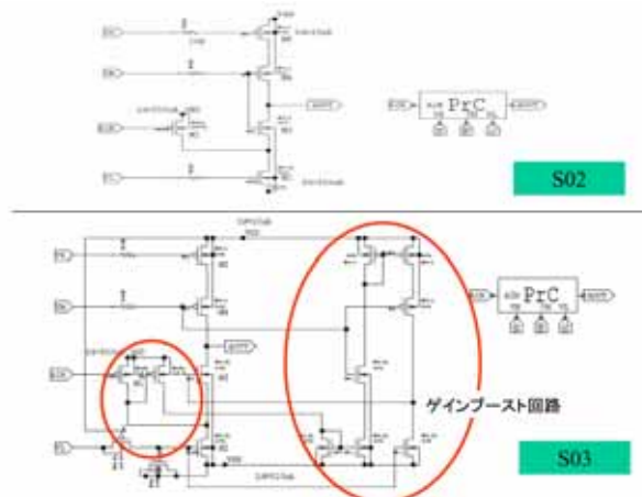
図 4.5: S02、S03 における前置増幅器回路
