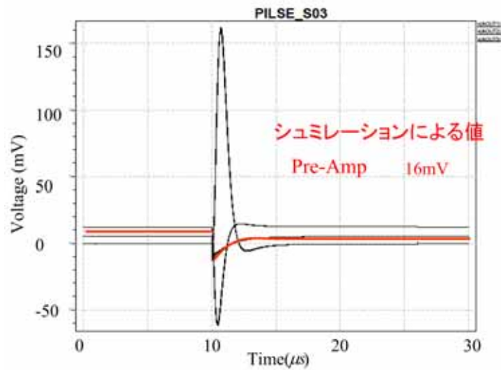
図 4.22: S03:前置増幅器シミュレーション
